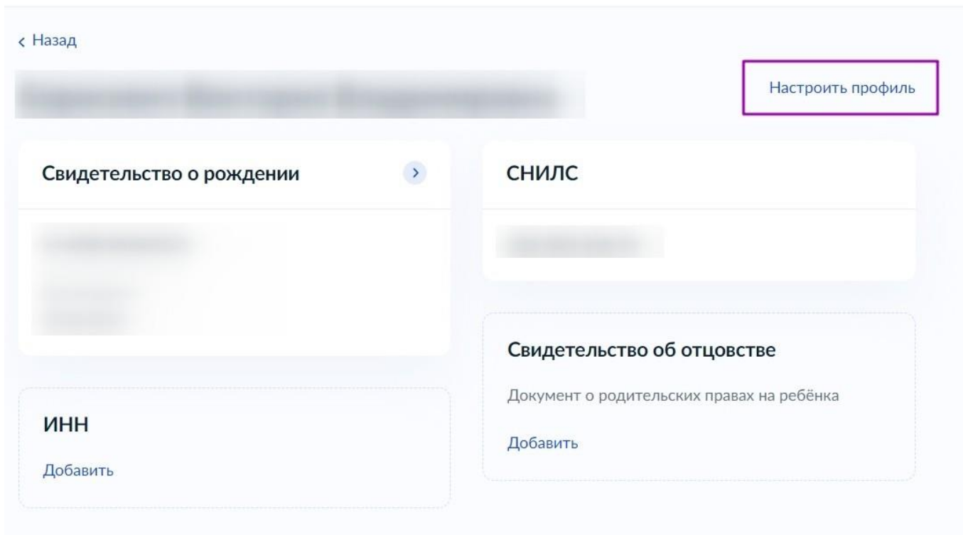
Рисунок 17. Настройка профиля
